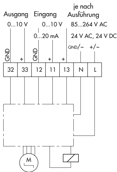
Bild 3: Elektrischer Anschluss
