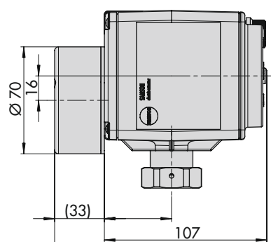
Bild 4: Maße in mm und Einbaulage
